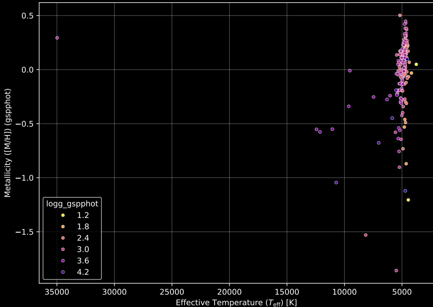
APOGEE DR17 Field: [020-06] Stellar Population Parameters (n= 225)
